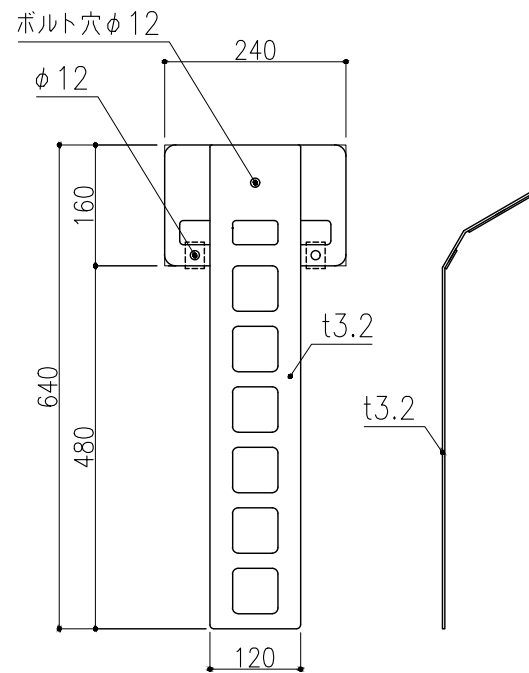
7.根鉢ロックピン S=1:3
