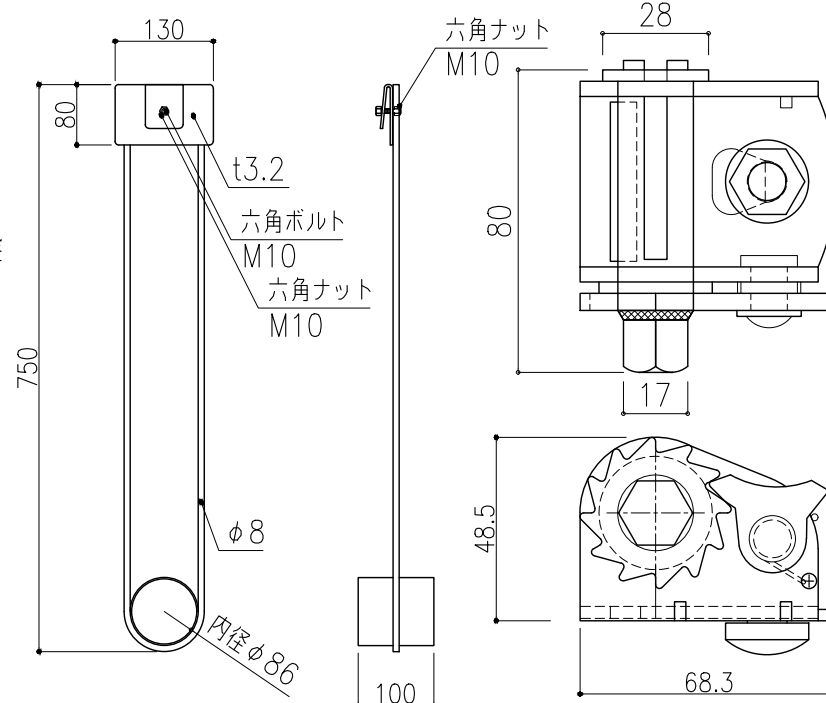
3.高さ調整型引上げアジャスター S=1:10 5.ベルトウィンチ S=1:2
