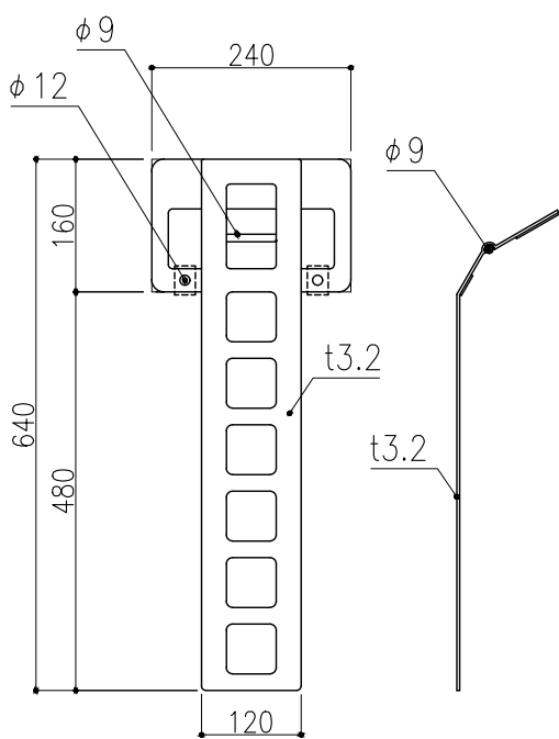
6.可動金具付幹巻ベルト S=1:3
