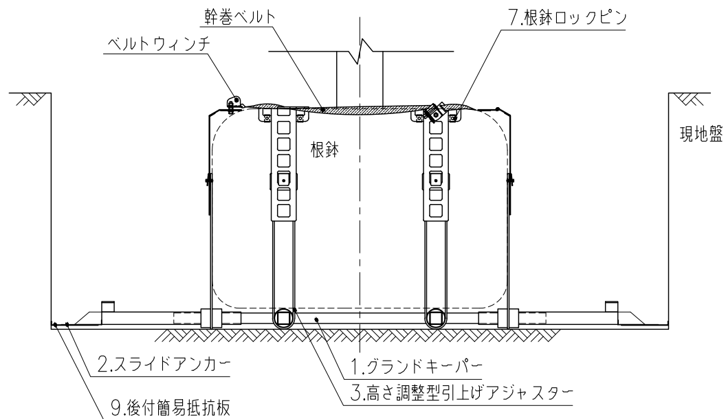
施工断面図 S=1:25
