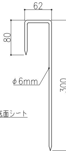
2.ピン S=1:5
