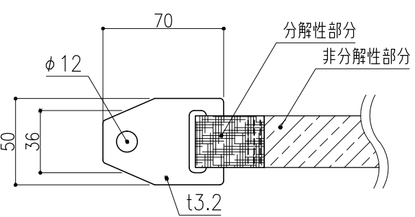
6.可動金具付幹巻ベルト S=1:3
